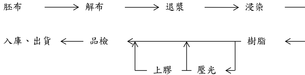
長織布染整生產流程
