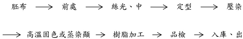
短織布染整生產流程
